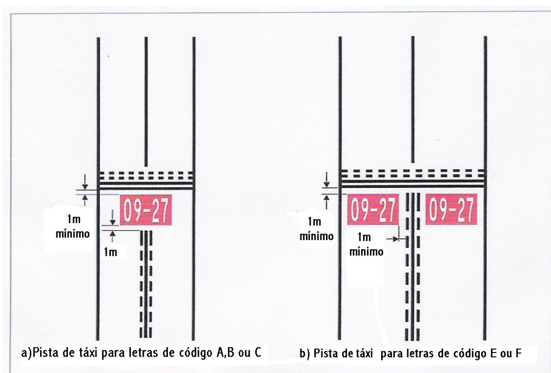
Figura D-9 Sinalização horizontal de instrução obrigatória
