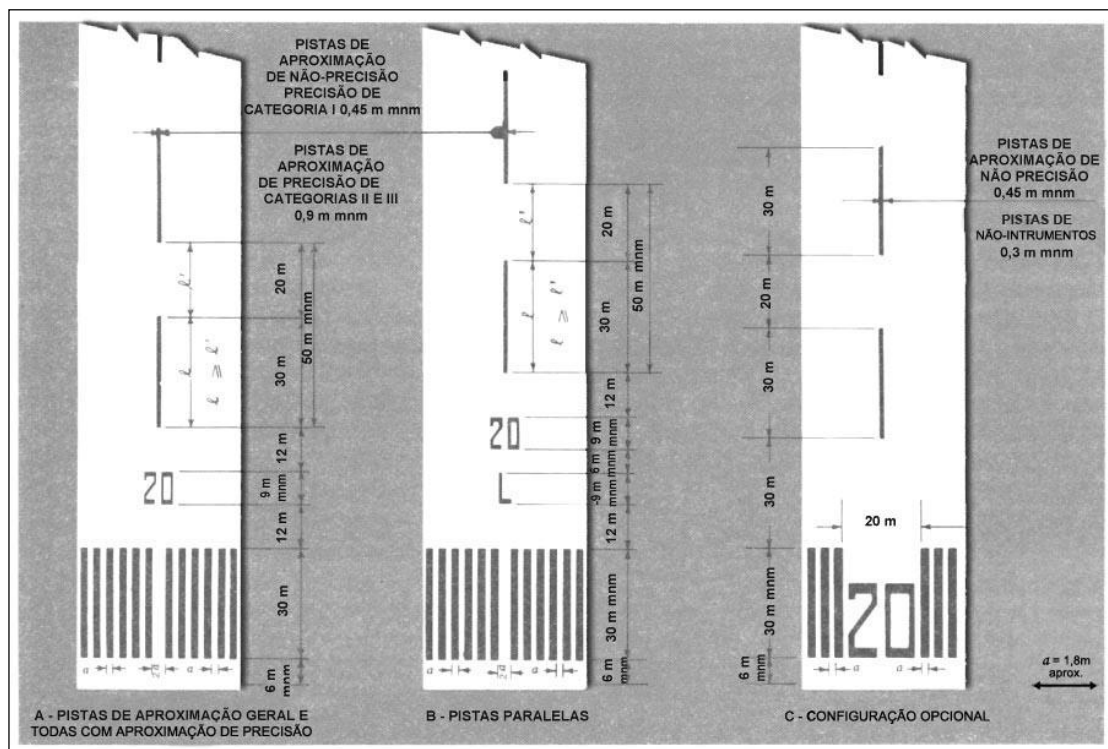
Figura D-2. Sinalização horizontal de designação de pista de pouso e decolagem, de eixo e cabeceira
