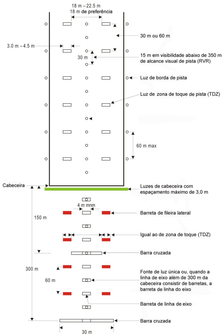
Figura D-14. 300 m mais internos de luzes de aproximação e luzes de pista de pouso e decolagem para aproximação de precisão Categorias II e III, onde os níveis de qualidade de serviço das luzes, especificados como objetivos de manutenção em 154.907 podem ser demonstrados.
