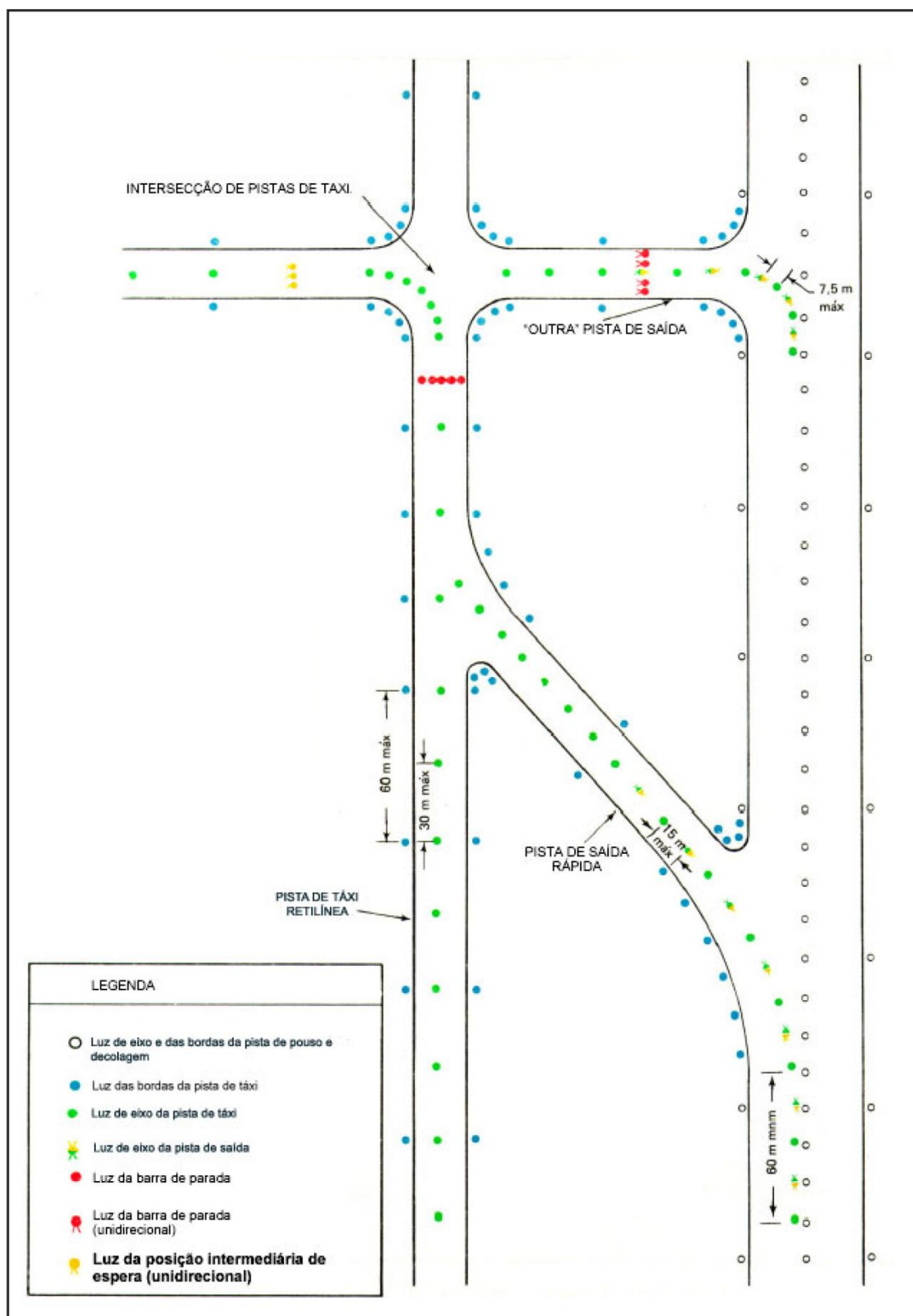
Figura D-24. Luzes de pista de taxi
