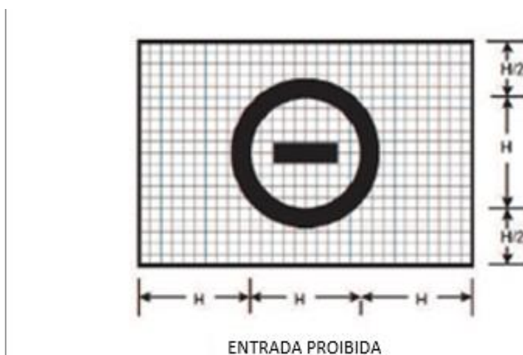
Sinalização vertical de “NO ENTRY” (NÃO ENTRE) (Alterado pela Resolução nº XXX, de DD.MM.AAAA)
