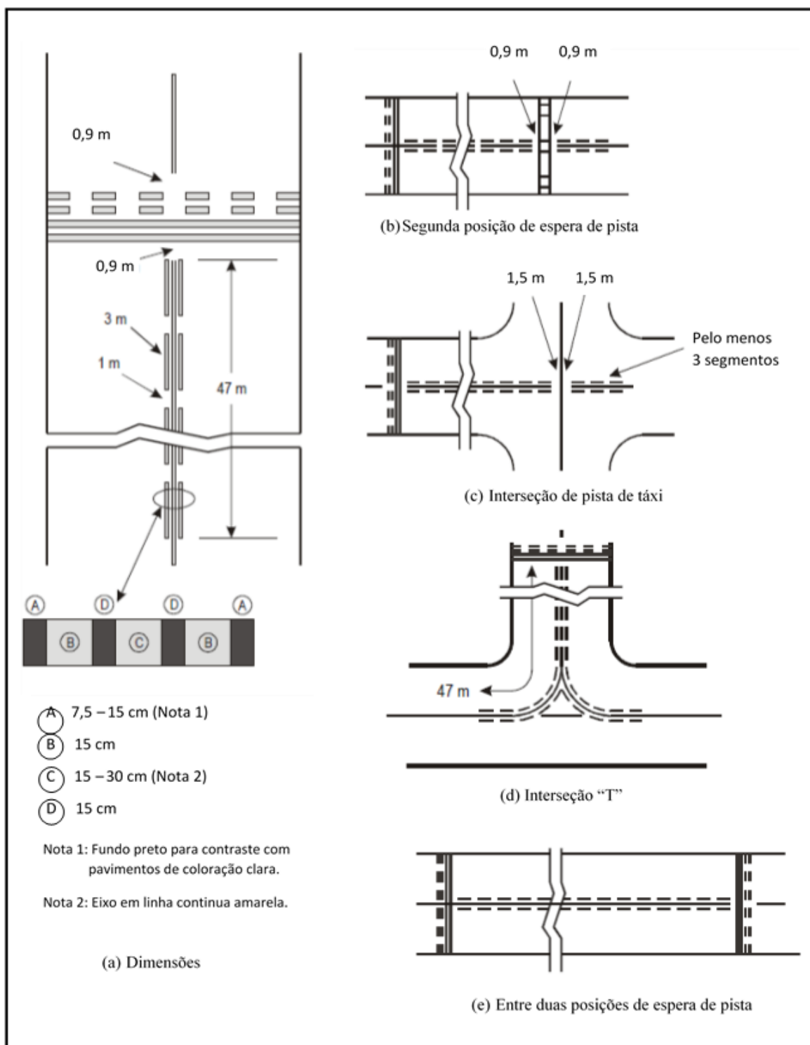
Figura D-6A - Sinalização horizontal melhorada de eixo de pista de táxi. (Alterado pela Resolução nº XXX, de DD.MM.AAAA)
