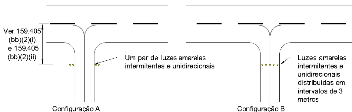
Figura D-26. Luzes de proteção de pista de pouso e decolagem (Alterado pela Resolução nº XXX, de DD.MM.AAAA)
