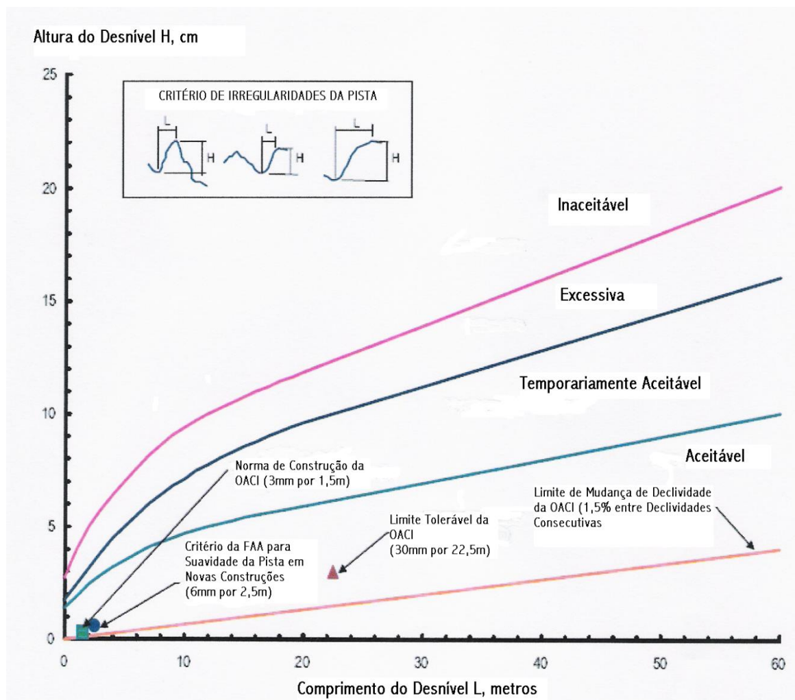
Figura AG-3. Critérios de irregularidade da superfície de uma pista (Numerado pela Resolução nº XXX, de DD.MM.AAAA)
