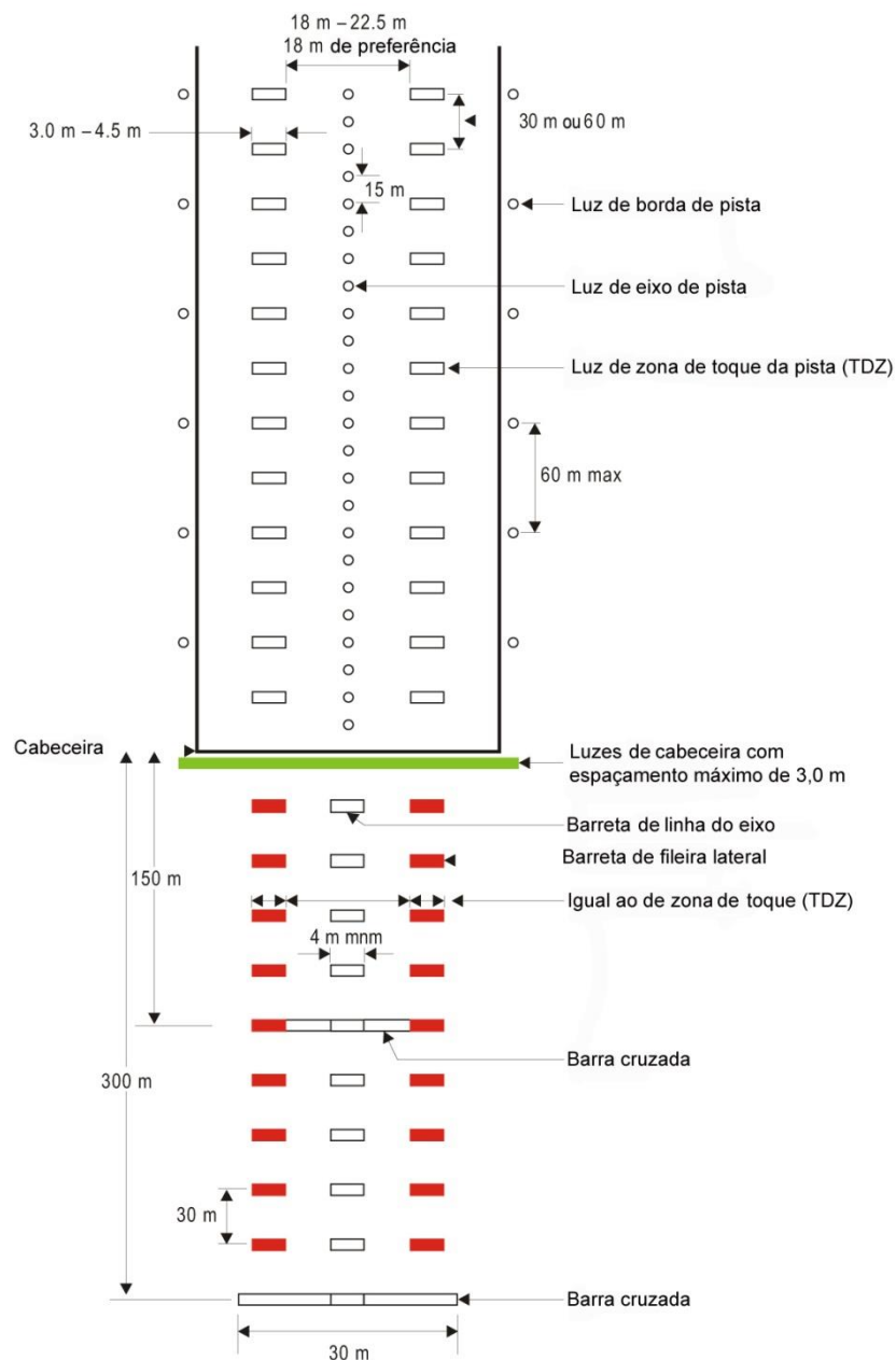
Figura D-13. 300 m mais internos de luzes de aproximação e luzes de pista de pouso e decolagem para aproximação de precisão Categorias II e III.
