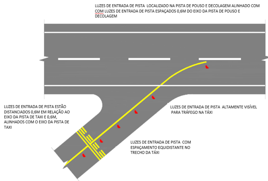
Figura D-26A. Luzes de situação de pista com táxi perpendicular
