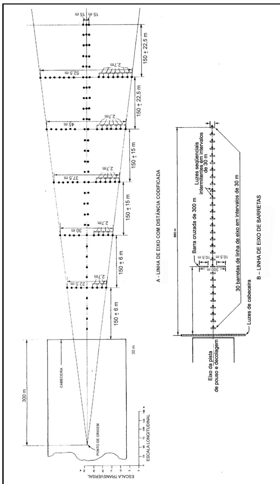
Figura AG-6. Sistema de luzes de aproximação de precisão categoria I
