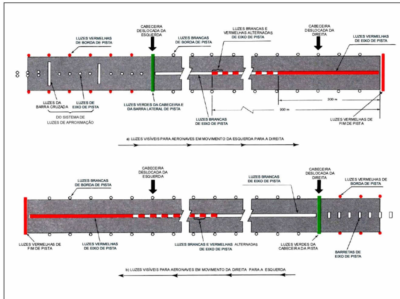
Figura D-22. Exemplo de luzes de aproximação e luzes de pista de pouso e decolagem em pistas com cabeceira deslocada
