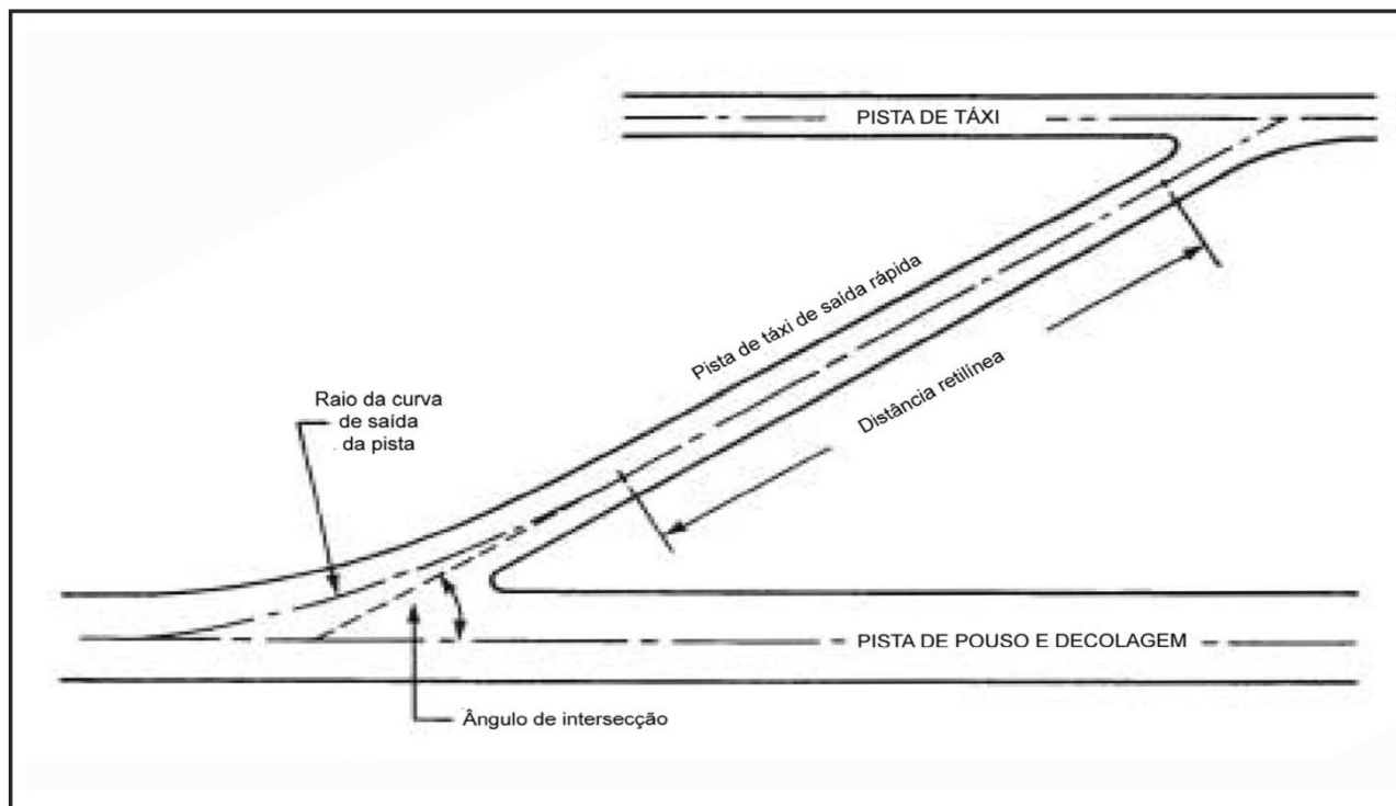
Figura C-3. Pista de táxi de saída rápida
