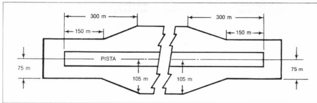
Figura C-2 – Parte nivelada de uma faixa de pista, incluindo uma pista de aproximação de precisão onde o número de código é 3 ou 4. (Incluído pela Resolução nº XXX, de DD.MM.AAAA)
