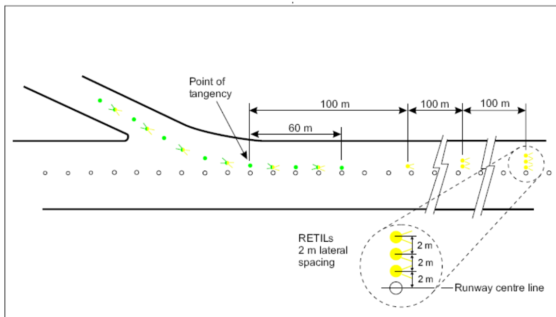
Figura D-23 Luzes da pista de táxi de saída rápida
