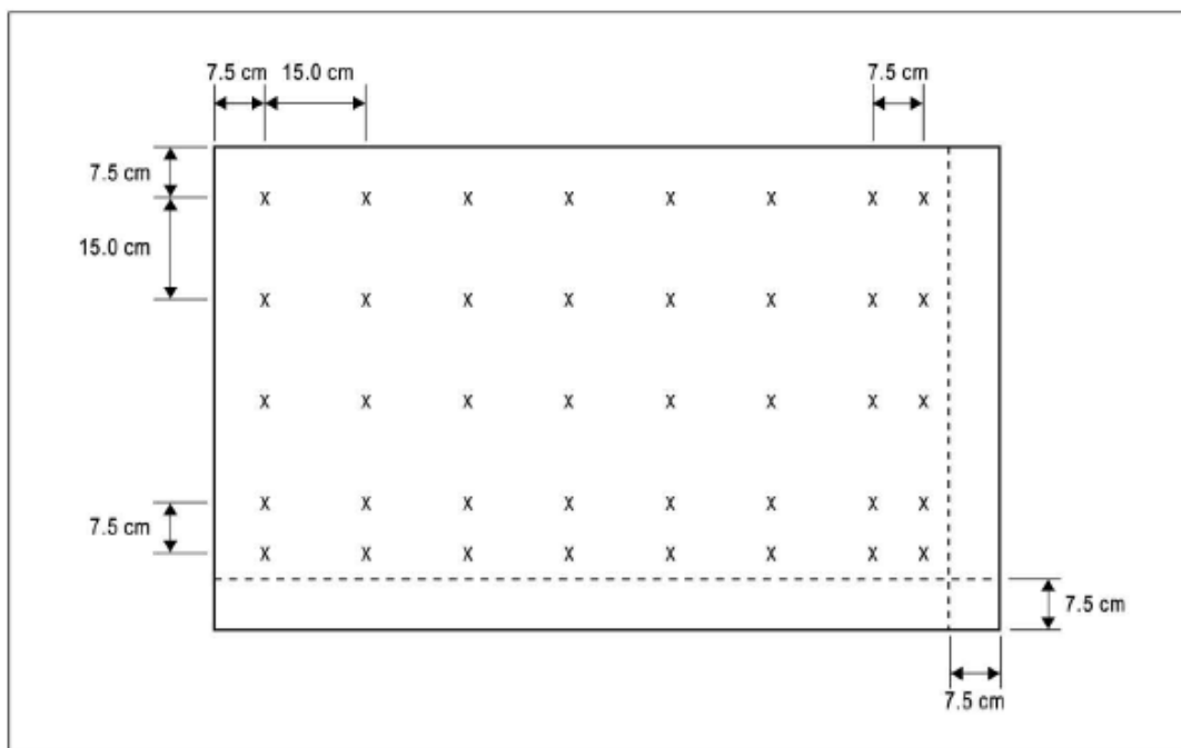
Figura AD-1. Pontos de coordenadas para calcular a luminância média de uma sinalização sertical
