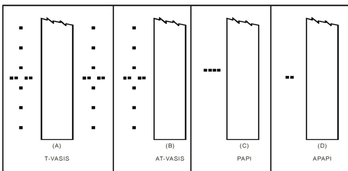
Figura D-15. Sistemas visuais indicadores de rampa de aproximação
