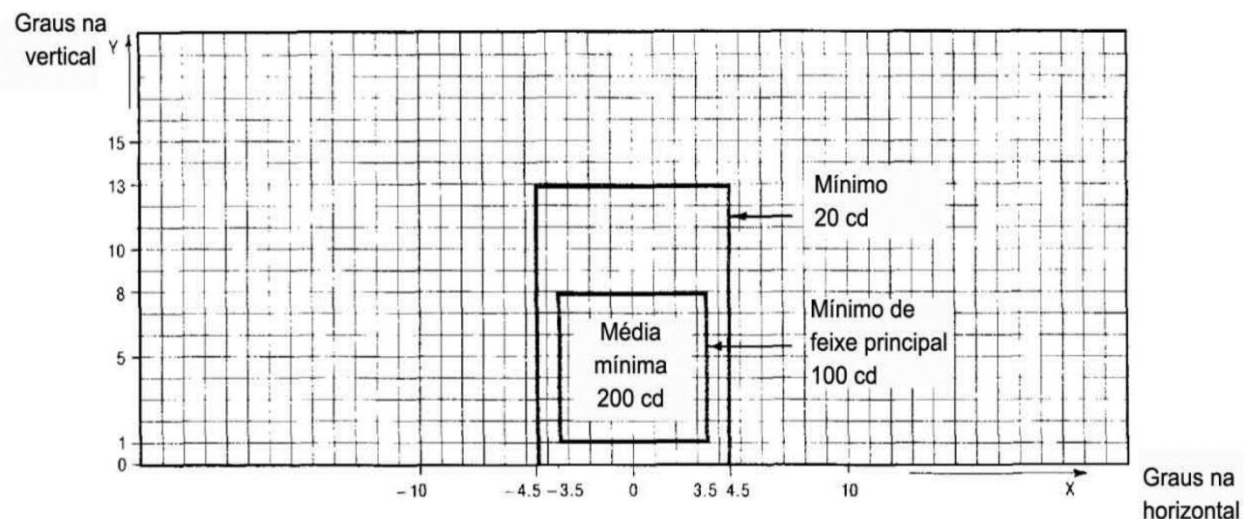
Figura AB-13. Diagrama de isocandela para as luzes do eixo da pista de táxi (espaçamento de 15 m) e de barras de parada em seções retas destinadas ao uso em condições de alcance visual da pista inferior a um valor de 350 m.
