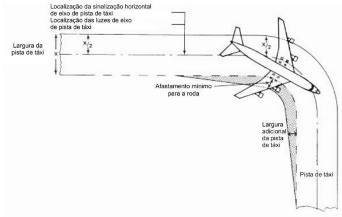
Figura C-2 Curvas de pista de táxi
