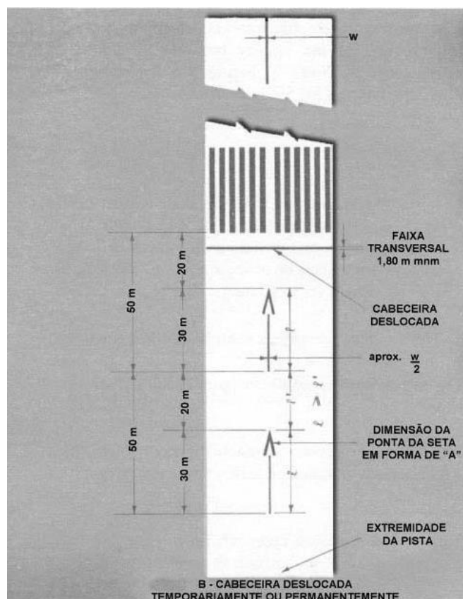
Figura D-4. Sinalização horizontal de cabeceira deslocada (Alterado pela Resolução nº XXX, de DD.MM.AAAA)
