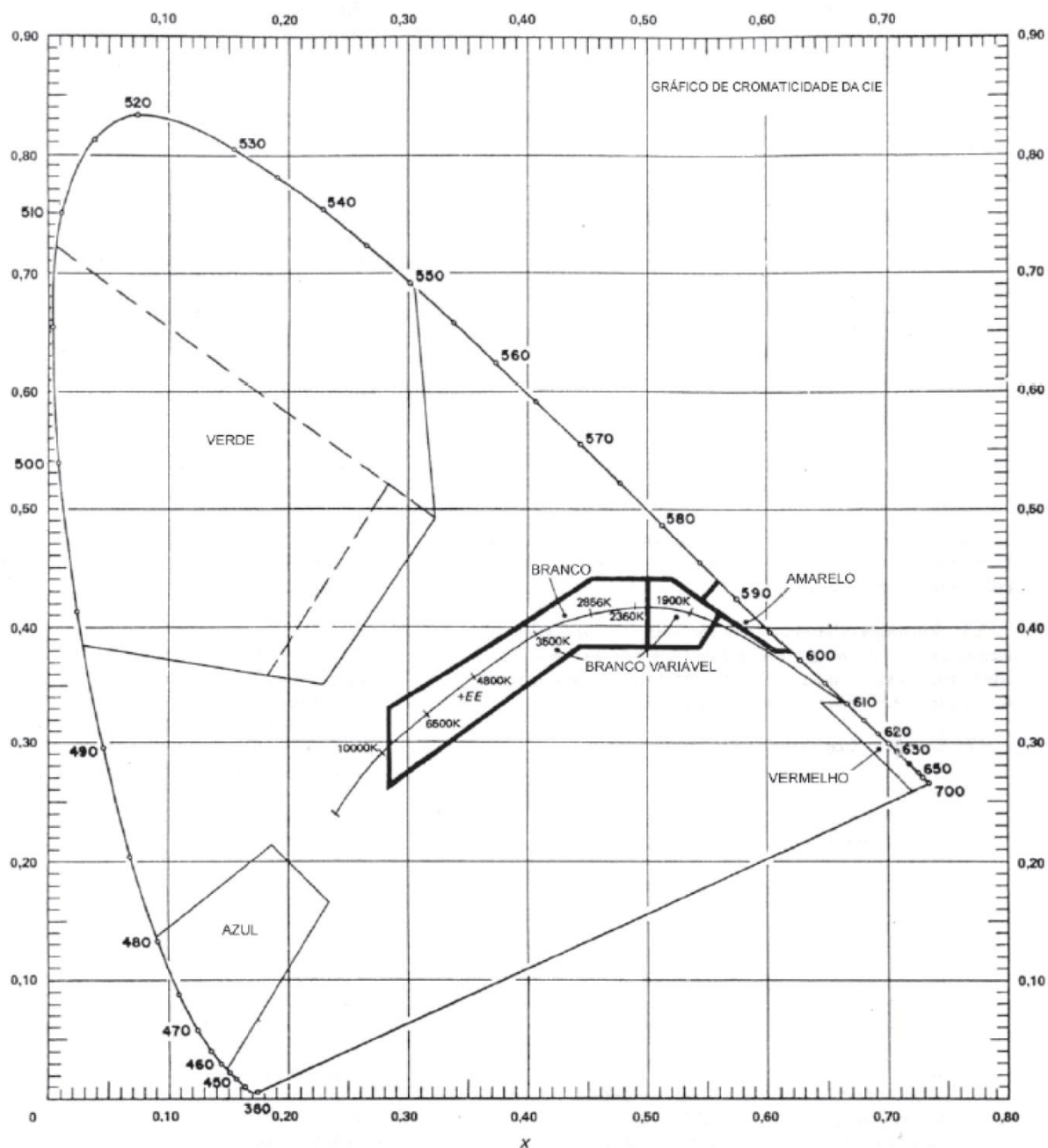
Figura AA-1. Cores para luzes aeronáuticas de superfície (lâmpadas tipo filamento) (Redação dada pela Resolução nº XXX, de DD.MM.AAAA)
