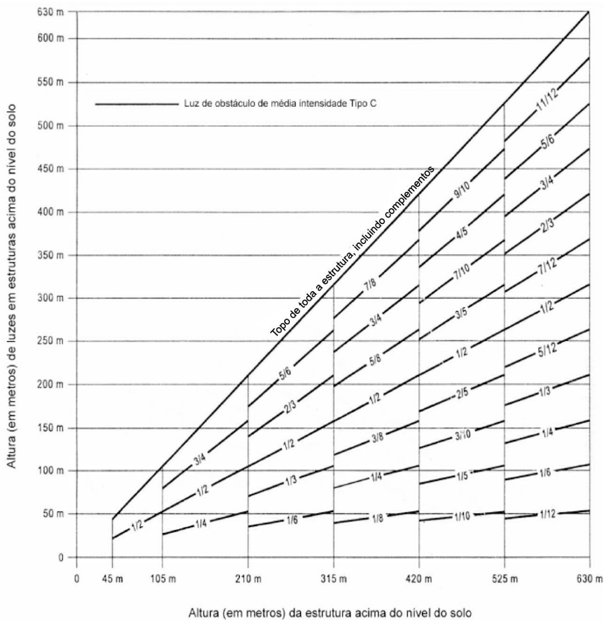
Figura AF-3. Sistema de iluminação de obstáculos de média intensidade com luzes vermelhas ininterruptas, Tipo C
