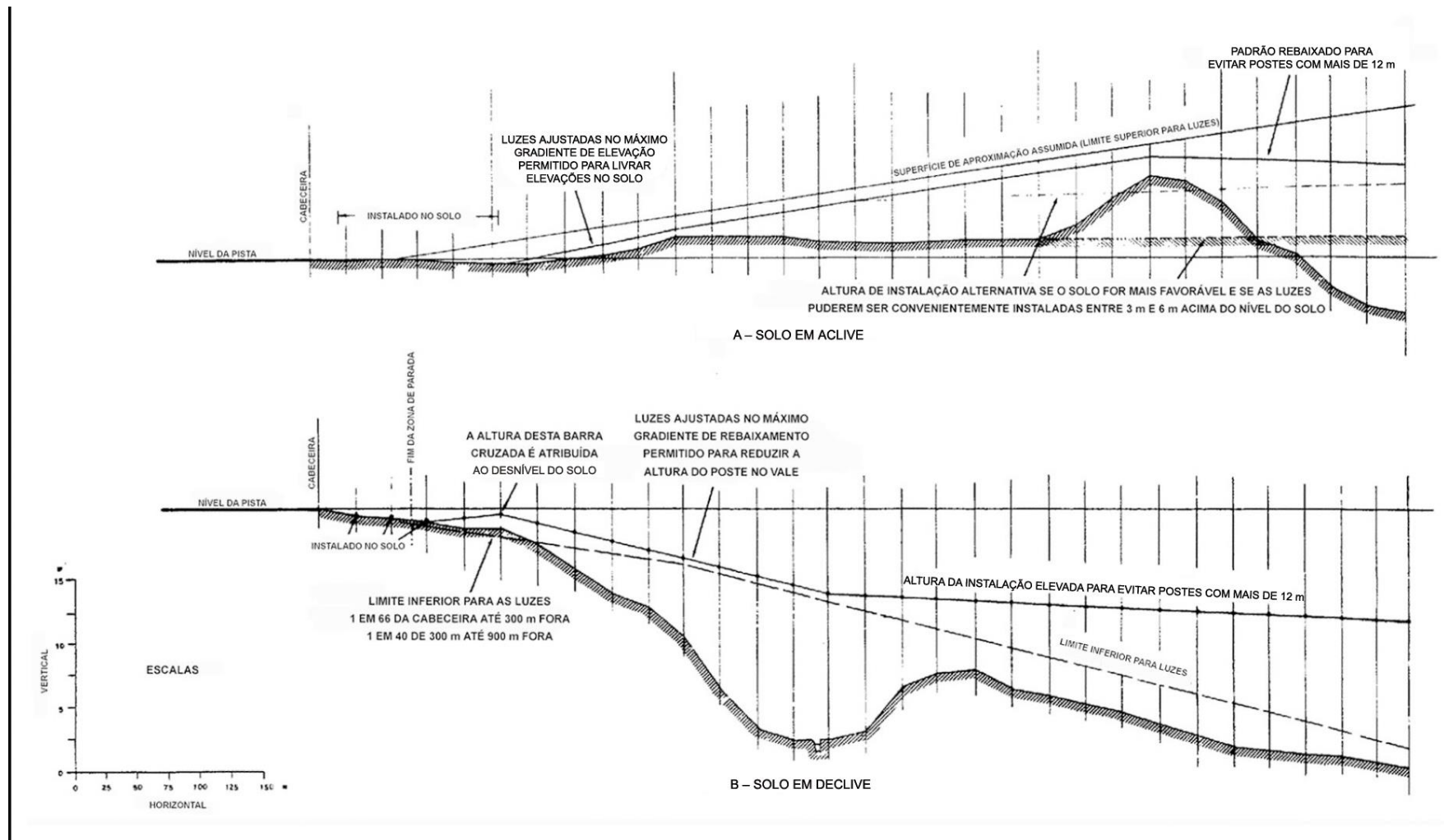
Figura AG-7. Tolerâncias verticais de instalações
