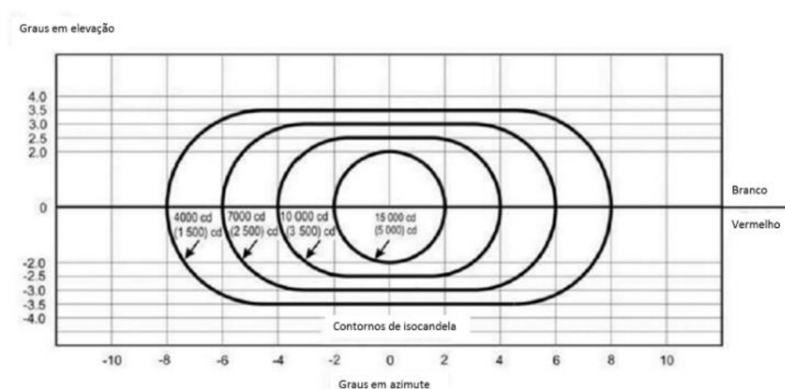
Figura AB-23. Distribuição da intensidade de luz do PAPI e do APAPI. (Incluído pela Resolução nº XXX, de DD.MM.AAAA)
