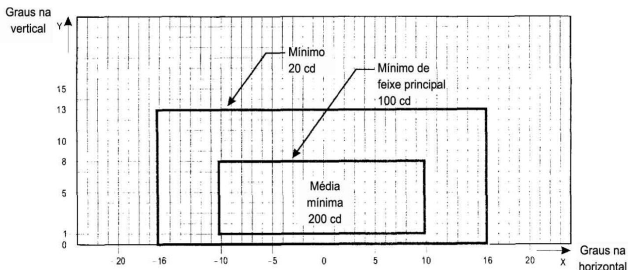
Figura AB-12. Diagrama de isocandela para as luzes do eixo da pista de táxi (espaçamento de 15 m) e de barras de parada em seções retas destinadas ao uso em condições de alcance visual da pista inferior a um valor de 350 m, onde podem ocorrer grandes correções, bem como para luzes de proteção de pista de baixa intensidade, configuração b.
