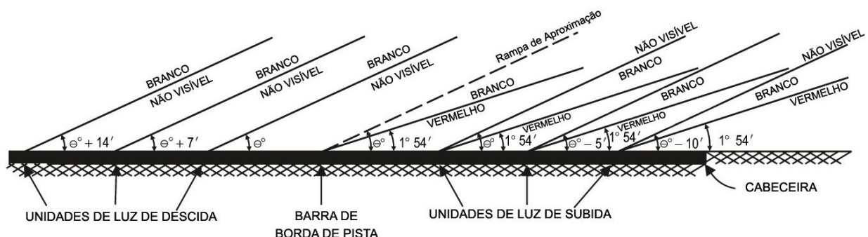
Figura D-17. Feixes de luzes e configurações de elevação do T-VASIS e AT-VASIS
