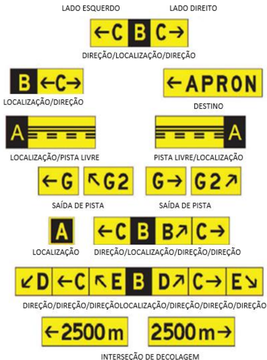
Figura D-28. Sinalizações verticais de informação (Alterado pela Resolução nº XXX, de DD.MM.AAAA)
