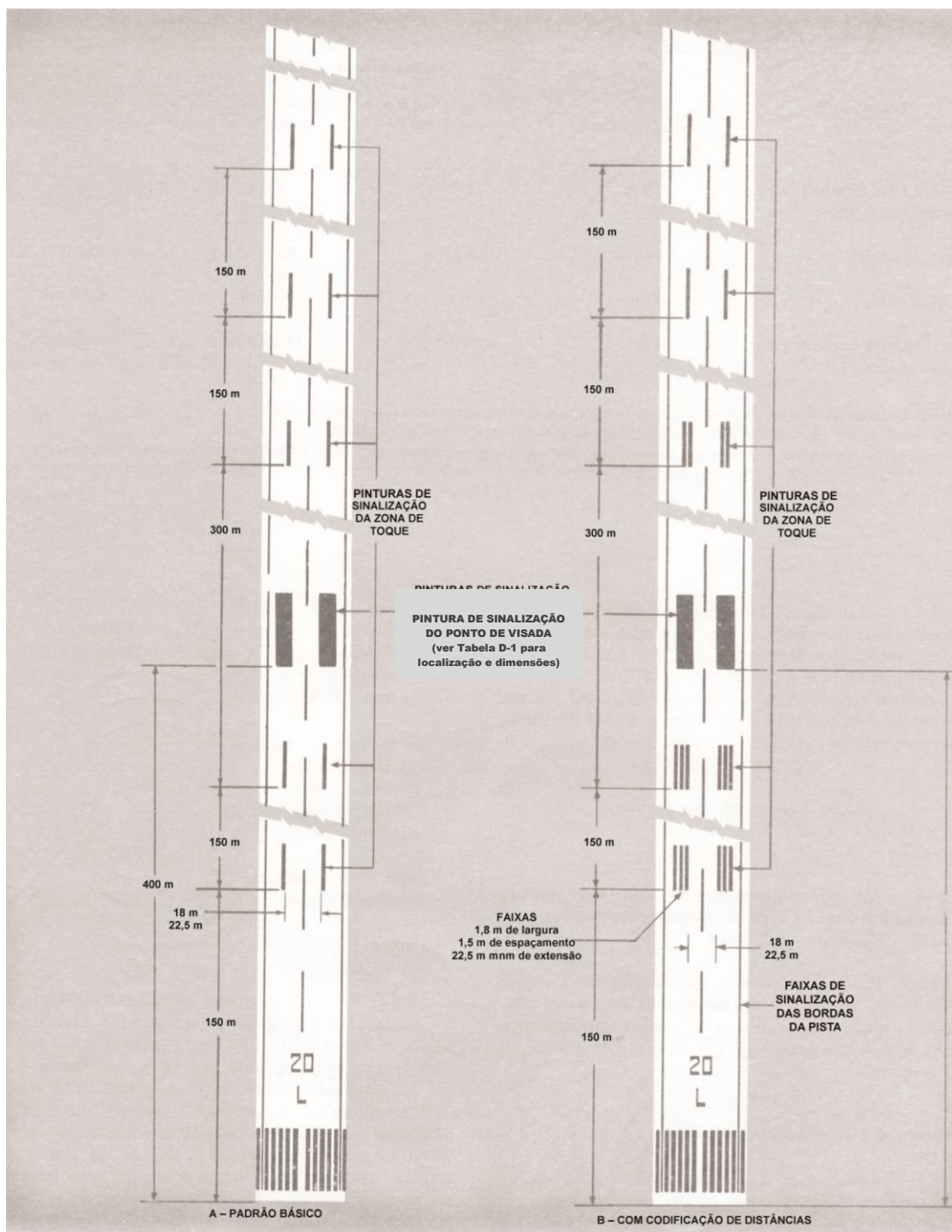
Figura D-5. Sinalização horizontal de ponto de visada e de zona de toque
