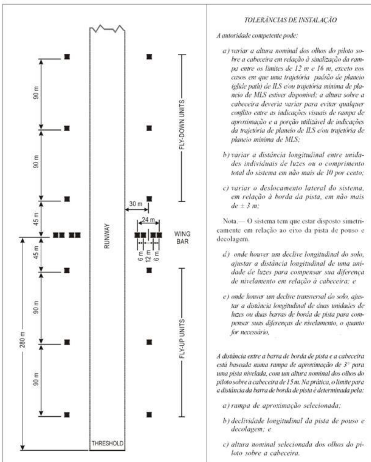
Figura D-16. Localização das unidades de luz para o T-VASIS
