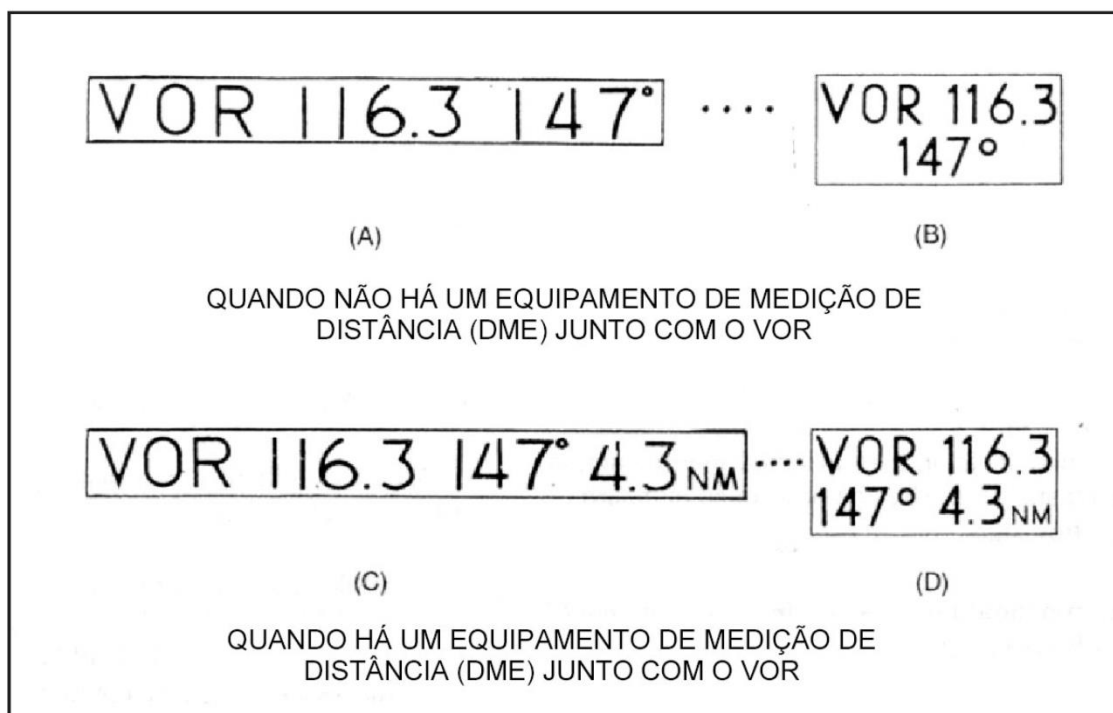
Figura D-30. Sinalizações verticais de ponto de teste de VOR de aeródromo.
