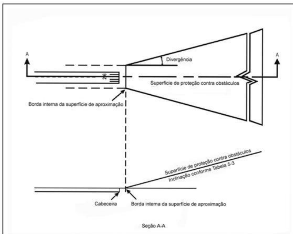
Figura D-20. Superfície de proteção contra obstáculos para sistemas visuais indicadores de rampa de aproximação
