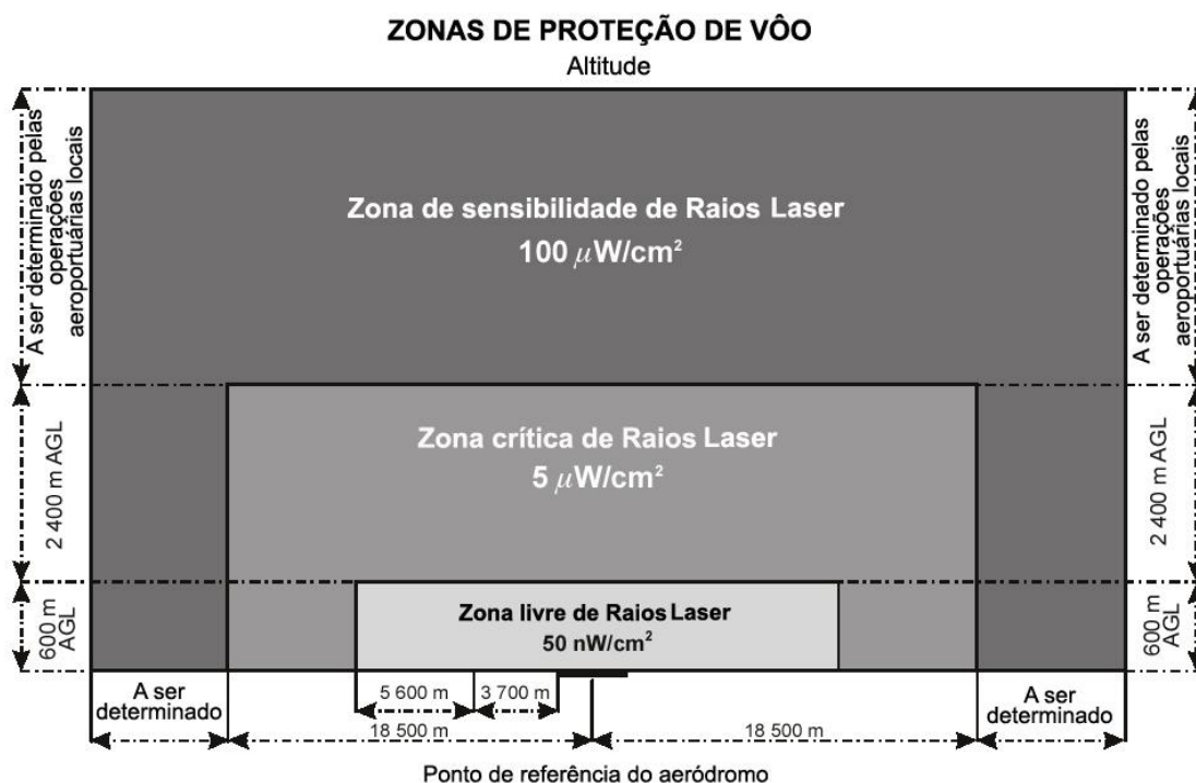
Figura D-12 – Zonas de proteção de voo com os níveis máximos de irradiação para raios laser visíveis.
