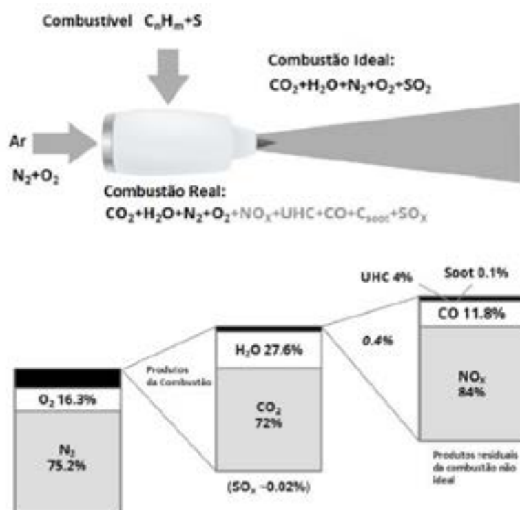
Figura 1: Desenho esquemático da combustão ideal e combustão real. Fonte: Adaptado de IPCC (1999).
