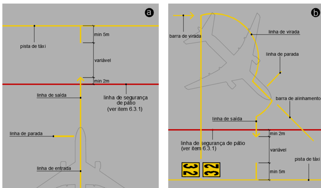
Figura 18 – Linha de saída descontínua com seta de indicação de continuidade
