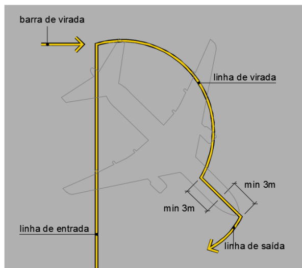
Figura 12 – Linha de virada
