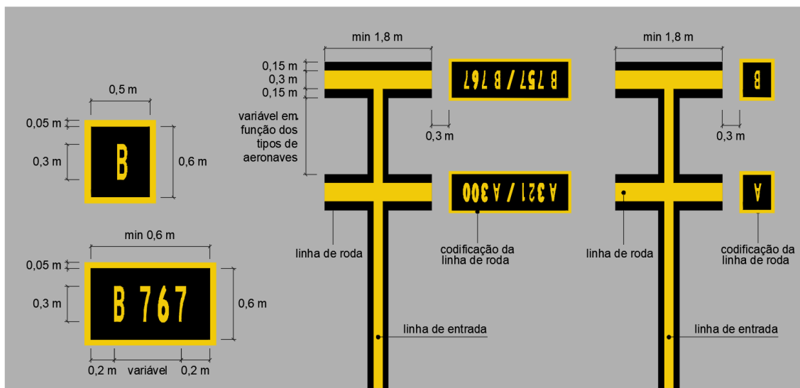
Figura 16 – Linhas de roda codificadas
