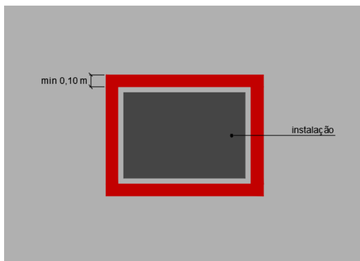
Figura 51 – Identificação de instalação de pátio
