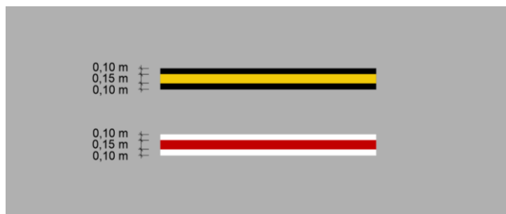
Figura 1 – Contornos em sinalizações horizontais de pátio de aeronaves
