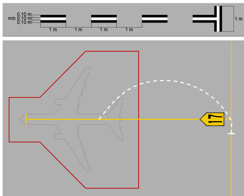
Figura 52 – Linha de guia de pushback
