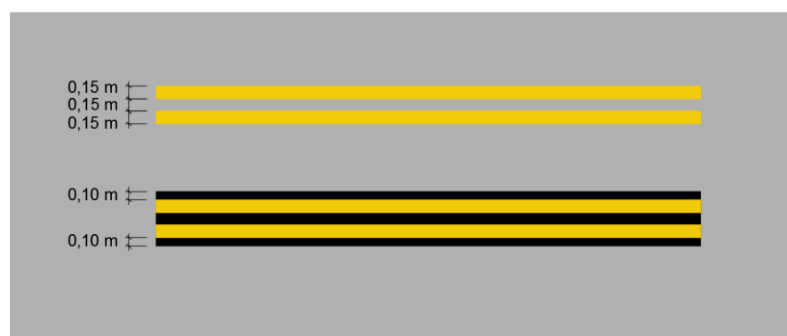
Figura 29 – Sinalização horizontal de borda de pátio de aeronaves
