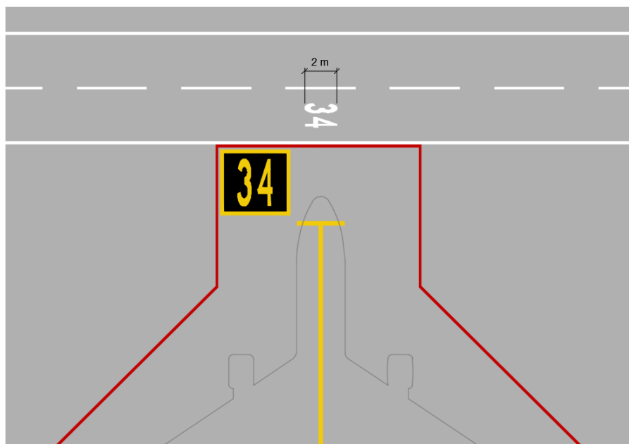
Figura 56 – Indicação de posição de estacionamento de aeronaves em via de serviço
