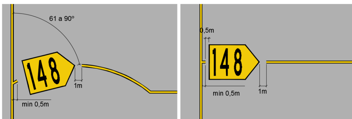
Figura 7 – Localização da identificação de posição de estacionamento (a) em relação à linha de entrada
