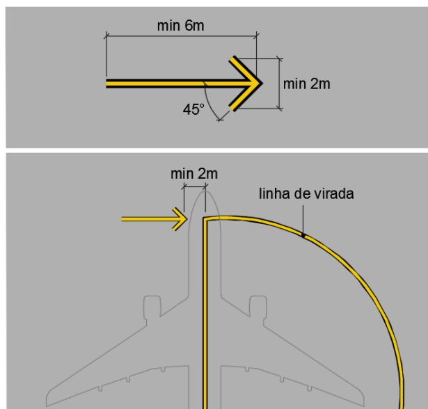
Figura 10 – Barra de virada
