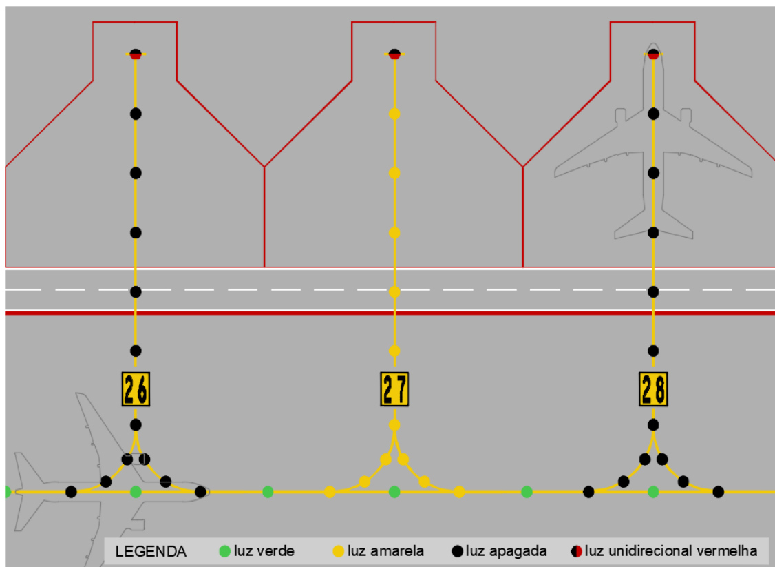
Figura 62 – Sistema de luzes de orientação de manobras de estacionamento de aeronaves
