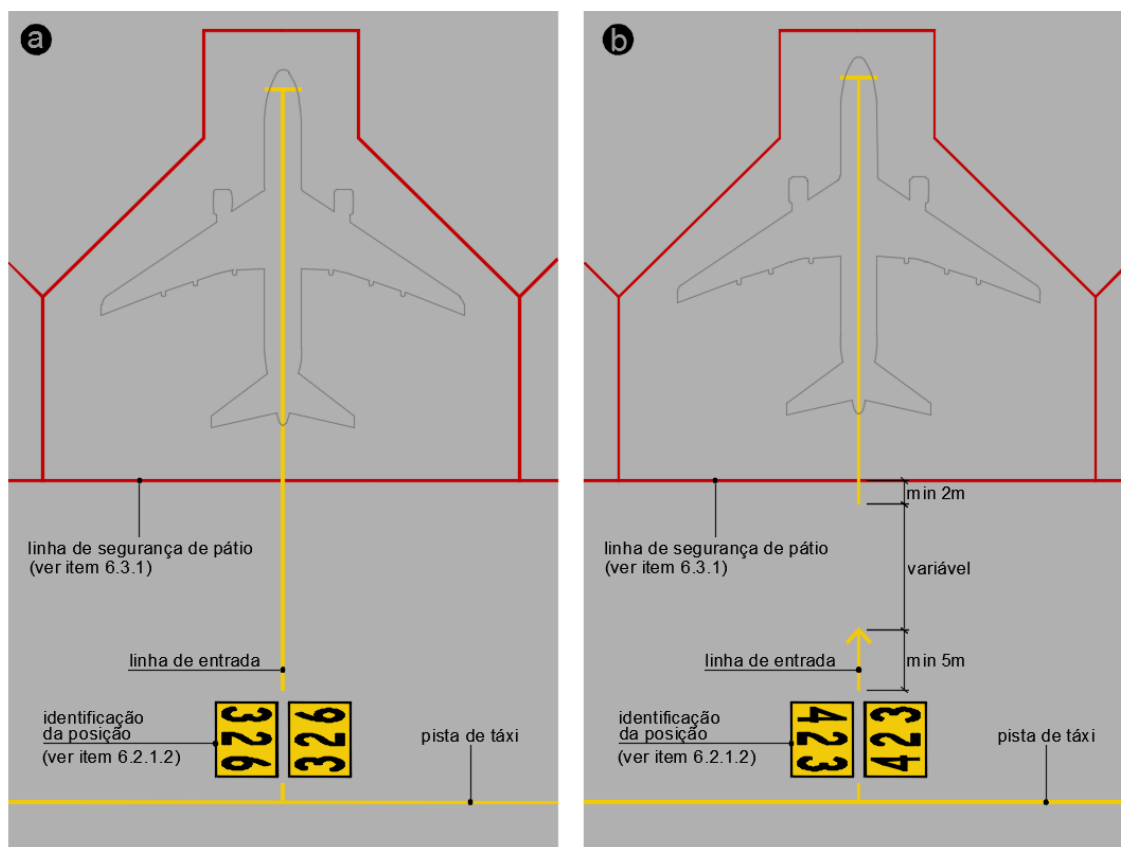
Figura 4 – Linha de entrada completa (a) e com seta de indicação de continuidade (b)
