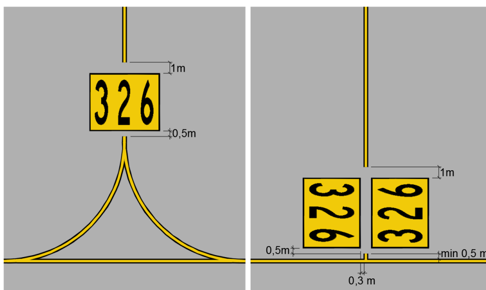
Figura 9 – Localização da identificação de posição de estacionamento (c) em relação à linha de entrada
