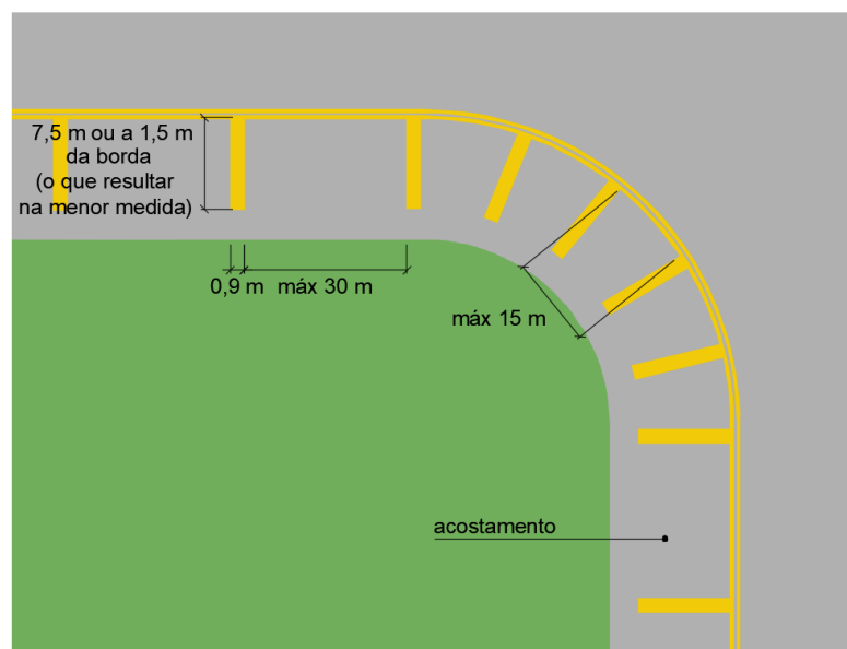
Figura 30 – Sinalização de acostamento de pátio sem capacidade de suporte
