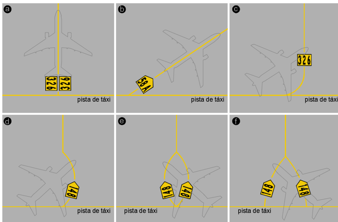
Figura 5 – Exemplos de linha de entrada
