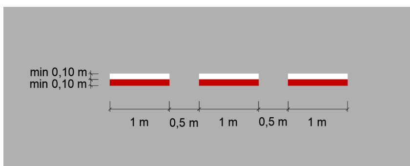
Figura 44 – Linha de restrição para áreas para posicionamento temporário de pessoas, veículos e equipamentos
