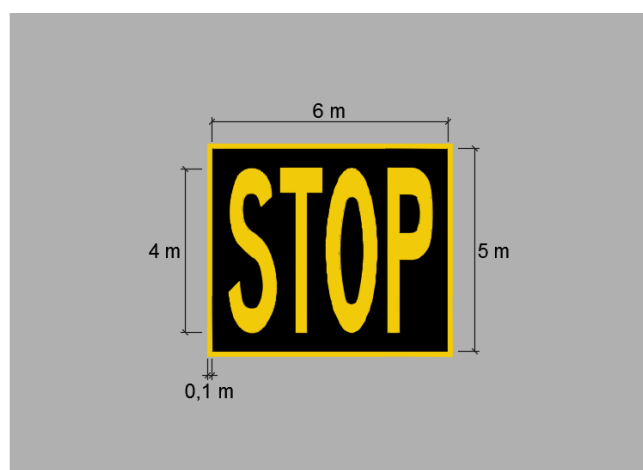
Figura 34 – Sinalização horizontal de localização de “STOP”
