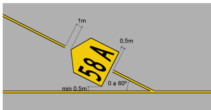
Figura 8 – Localização da identificação de posição de estacionamento (b) em relação à linha de entrada
