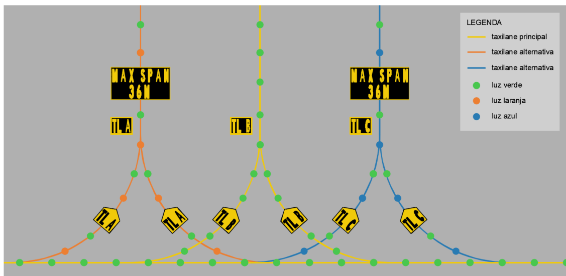
Figura 60 – Luzes de eixo de taxilanes alternativos
