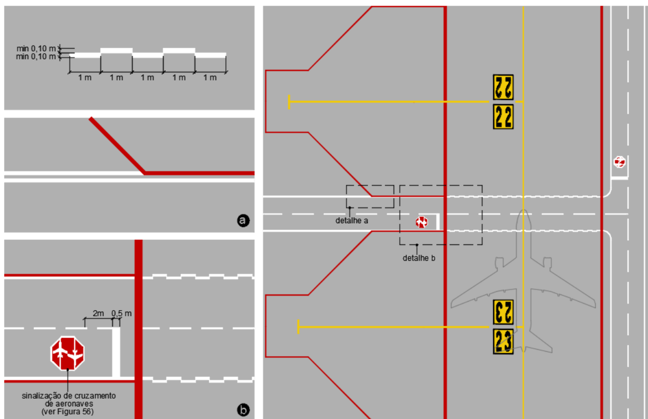
Figura 55 – Via de serviço em área de tráfego de aeronaves
