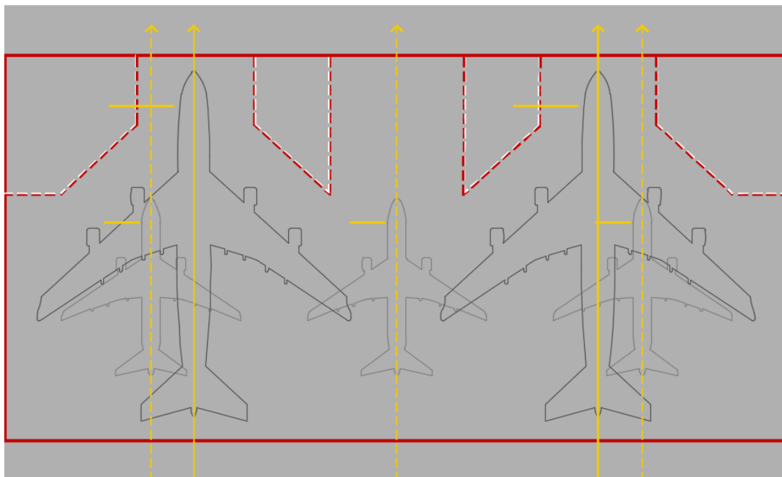
Figura 45 – Áreas para posicionamento temporário de pessoas, veículos e equipamentos
