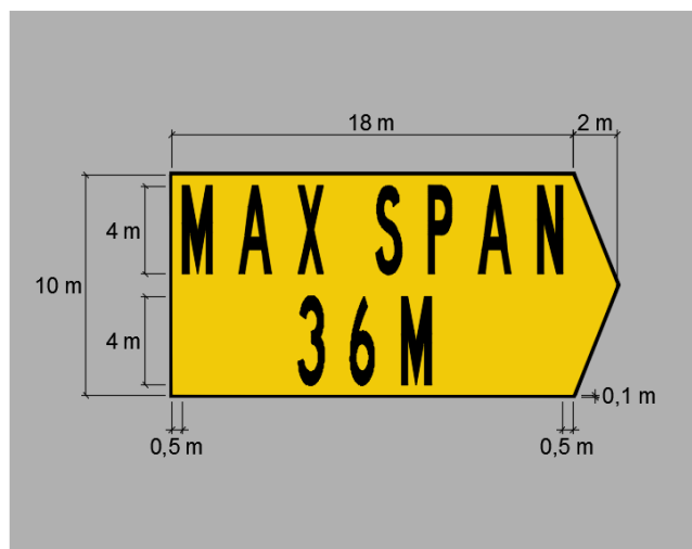
Figura 39 – Sinalização horizontal de direção de “MAX SPAN”
