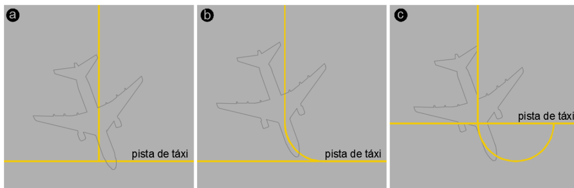
Figura 19 – Linha de saída (a) reta, (b) curva e (c) deslocada
