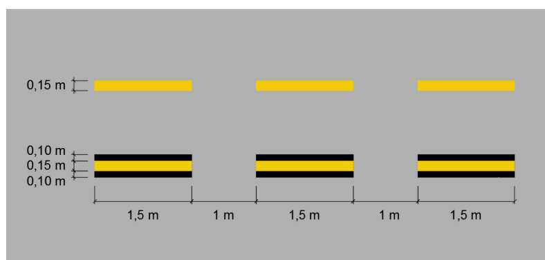
Figura 21 – Linhas interrompidas de entrada, virada e saída
