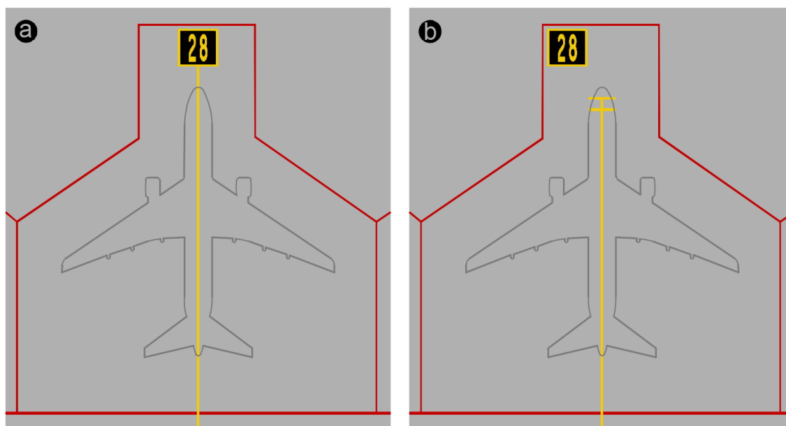
Figura 32 – Localização da sinalização de designação da posição de estacionamento sem linha de parada.
