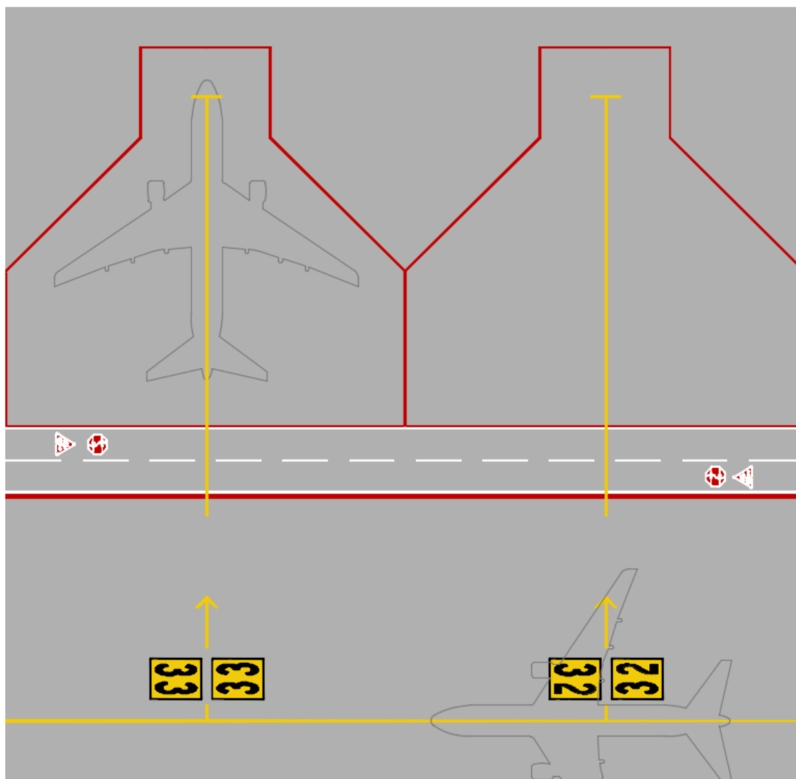
Figura 59 – Exemplo de uso das sinalizações horizontais de informação para motoristas de veículos e equipamentos
