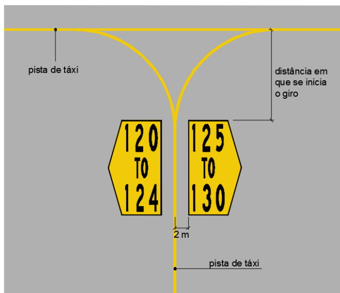
Figura 38 – Localização das sinalizações horizontais de direção de posição de estacionamento
