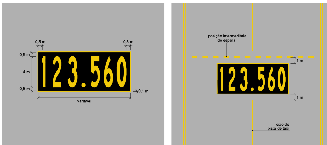
Figura 36 – Sinalização horizontal de frequência de comunicação
