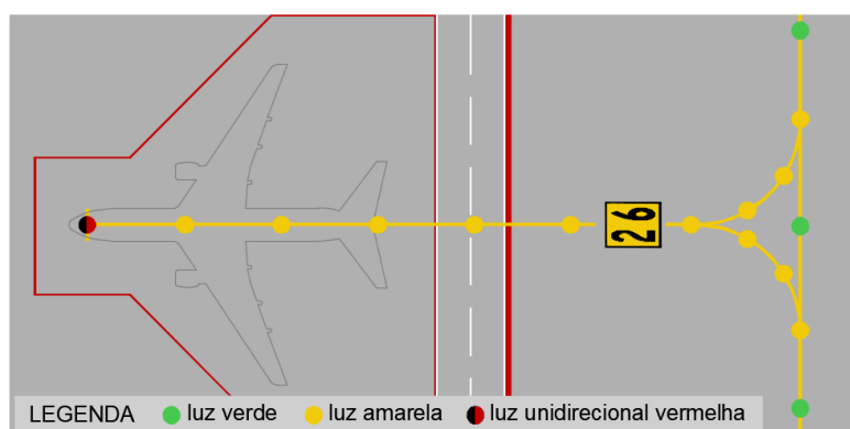
Figura 61 – Luzes de orientação de manobras de estacionamento de aeronaves
