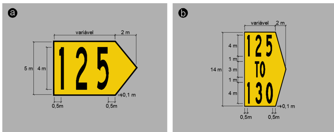
Figura 37 – Sinalizações horizontais de direção de posição de estacionamento
