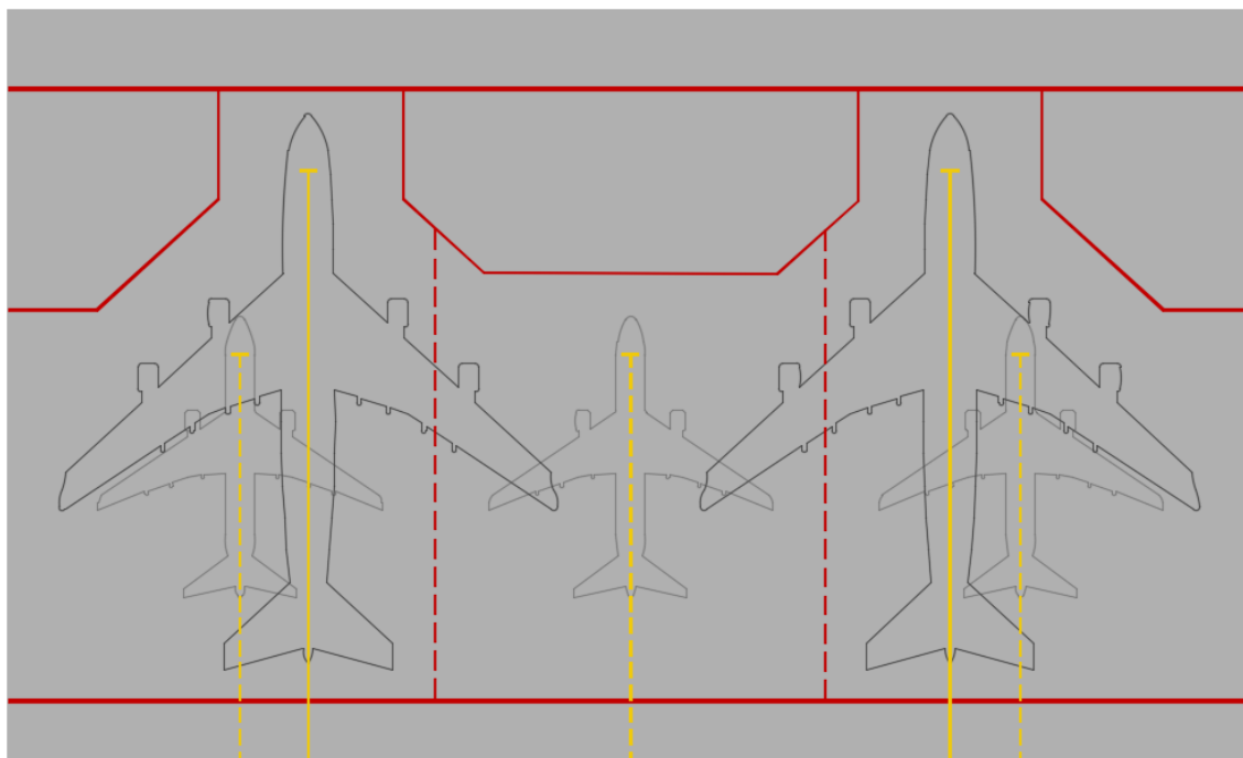
Figura 48 – Delimitação das áreas livres de pessoas, veículos ou equipamentos das posições de estacionamento secundárias
