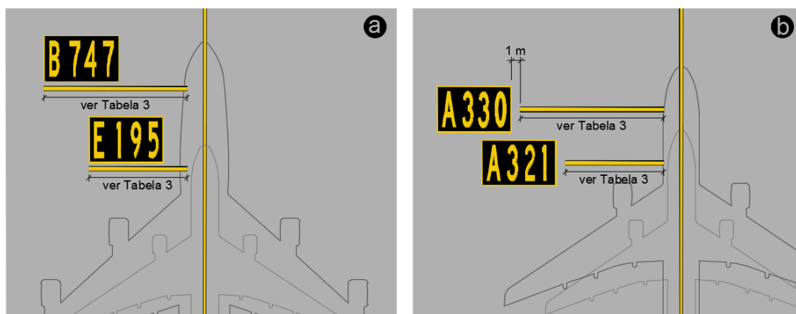
Figura 15 – Múltiplas linhas de parada codificadas
