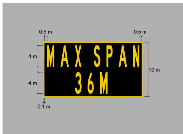
Figura 35- Sinalização horizontal de localização de "MAX SPAN"
