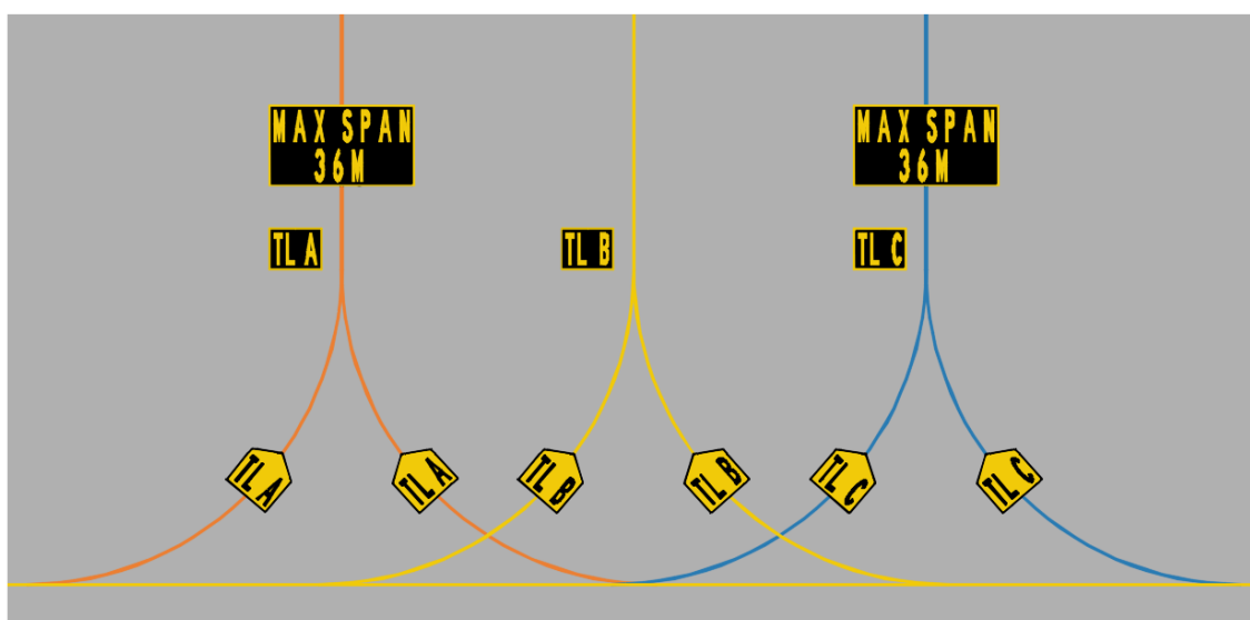
Figura 27 – Exemplo de utilização das cores laranja e azul e da sinalização de "MAX SPAN" para pistas de táxi alternativas de acesso às posições de estacionamento
