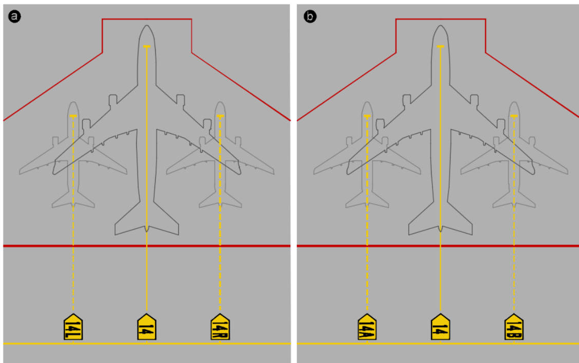
Figura 22 – Identificação de conjuntos de posição de estacionamento sobrepostos
