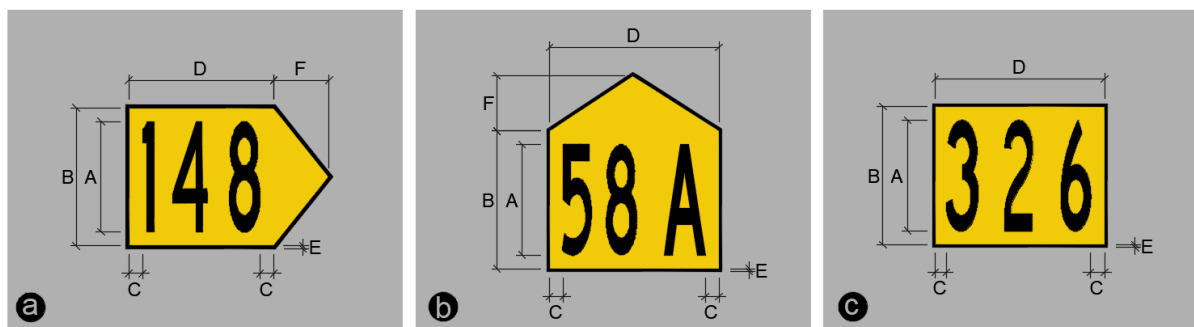
Figura 6 – Opções de sinalização horizontal de identificação de posição de estacionamento de aeronaves
