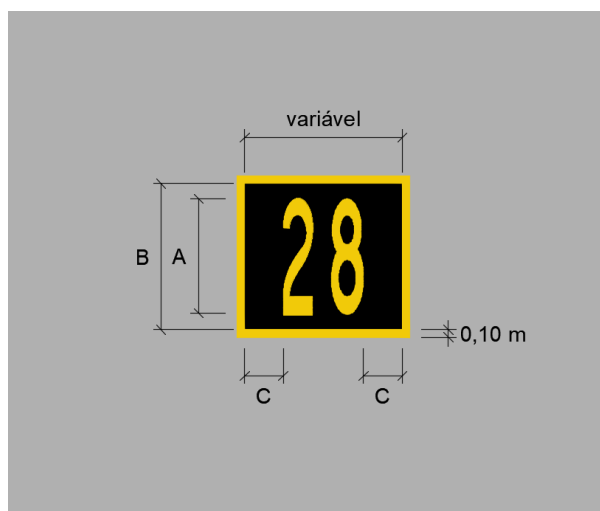
Figura 31 – Sinalização de designação da posição de estacionamento.
