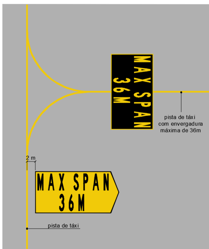
Figura 40 - Localização da sinalização horizontal de direção de “MAX SPAN”
