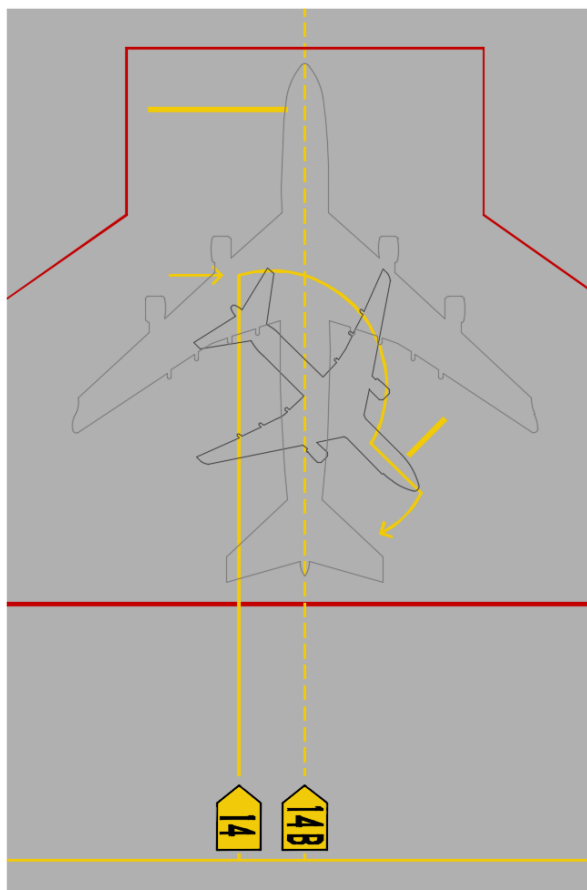
Figura 24- Exemplo de conjunto de posições de estacionamento sobrepostas
