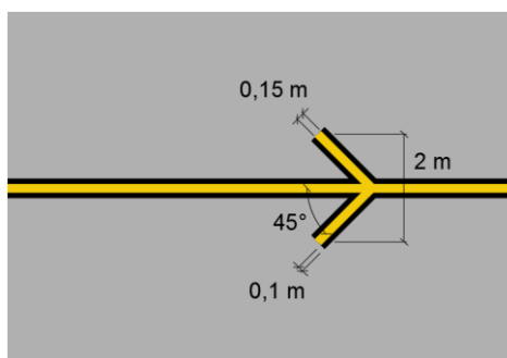
Figura 20 – Seta indicativa de direção única
