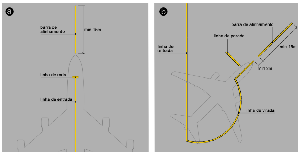
Figura 13 – Exemplos de utilização da barra de alinhamento
