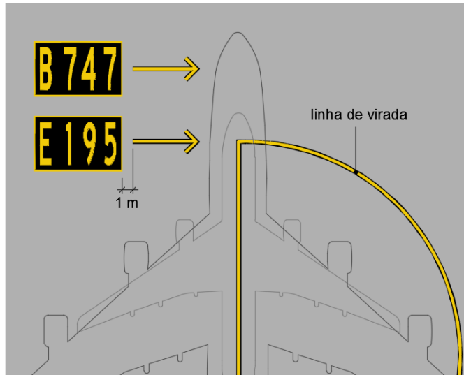
Figura 11 – Codificação de barras de virada
