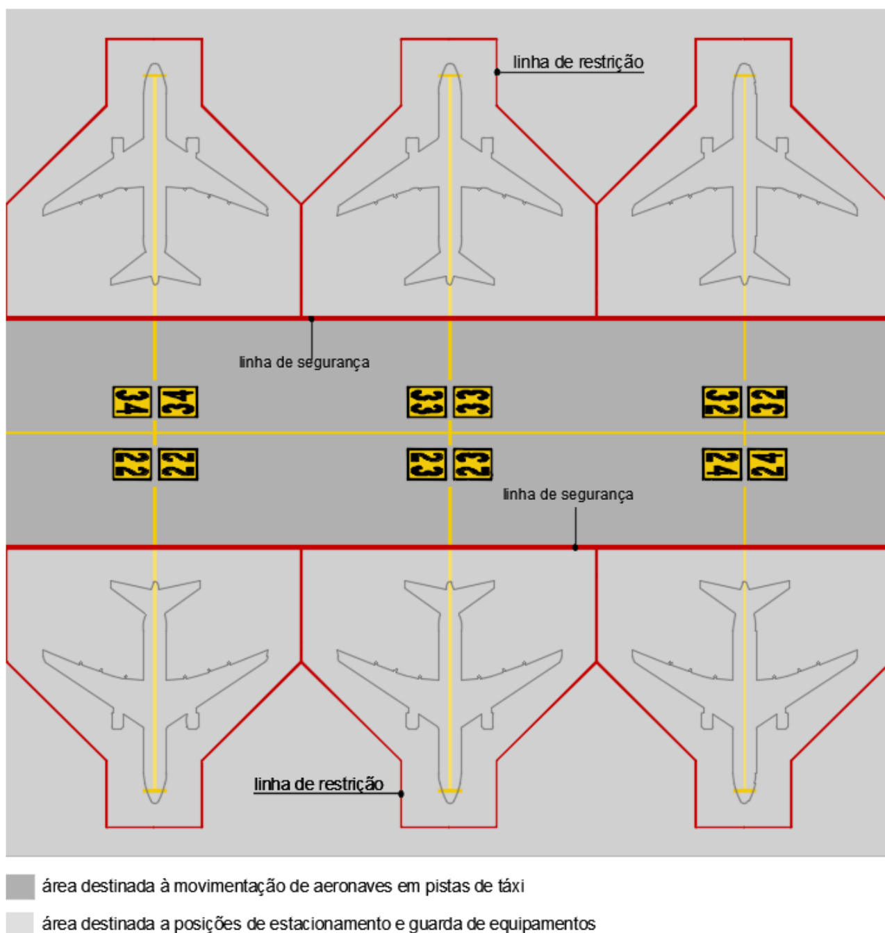
Figura 43 – Linhas de segurança de pátio
