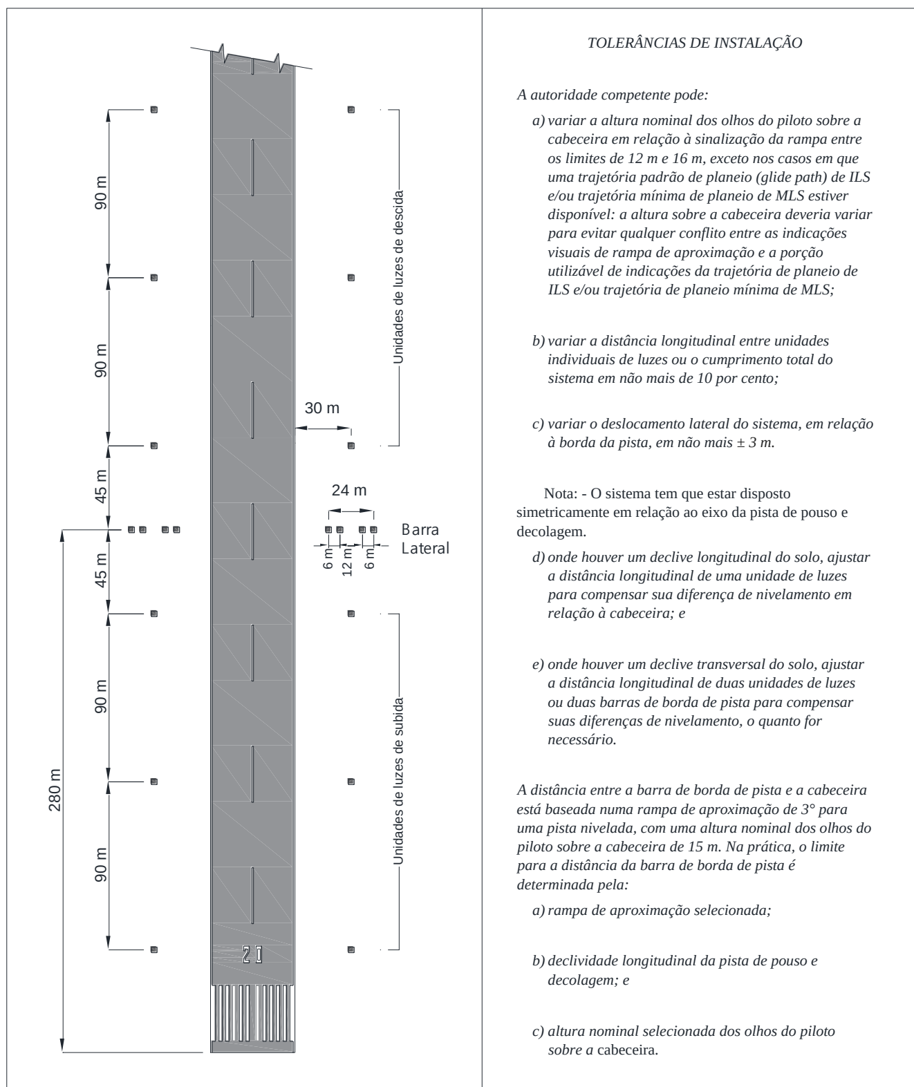
Figura D-13. Localização das unidades de luz para o T-VASIS
