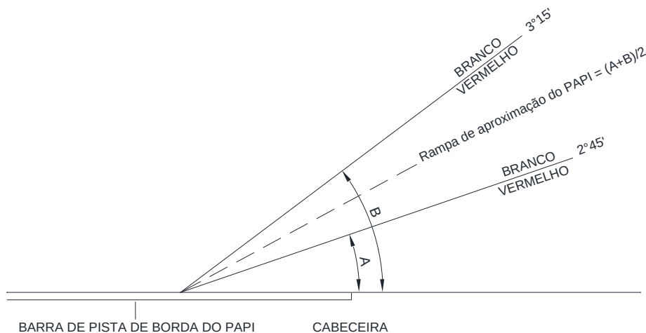
B - ILUSTRAÇÃO DO PAPI DE 3°
