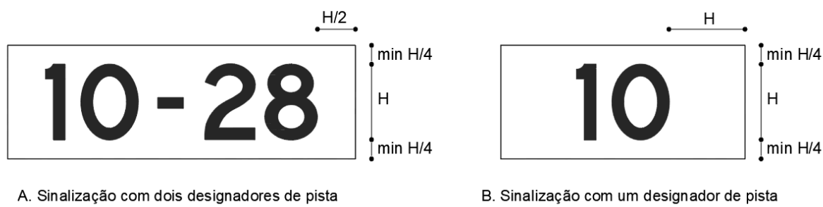
Figura AD-3. Dimensões das placas de sinalização vertical (Alterado pela Resolução nº 628, de 11.06.2021)
