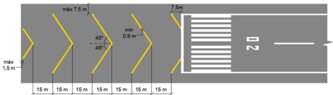
Figura E-2. Sinalização de área anterior à cabeceira (Alterado pela Resolução nº 628, de 11.06.2021)
