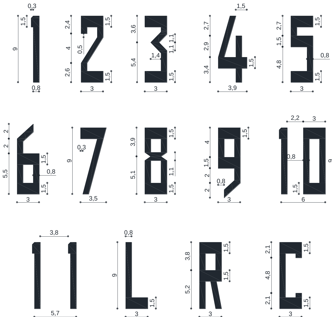
Figura D-3. Formato e proporções dos números e letras para sinalização horizontal de designação de pistas de pouso e decolagem (dimensões em m). (Alterado pela Resolução nº 465, de 13.03.2018)
