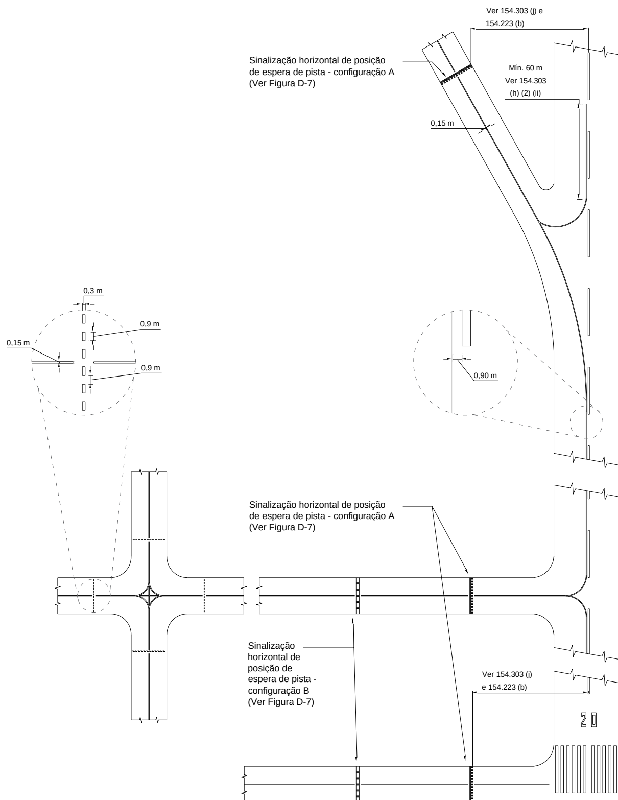
Figura D-6. Sinalização horizontal de pista de táxi (exibida em conjunto com a sinalização horizontal básica de pista de pouso e decolagem) (Alterado pela Resolução nº 465, de 13.03.2018)
