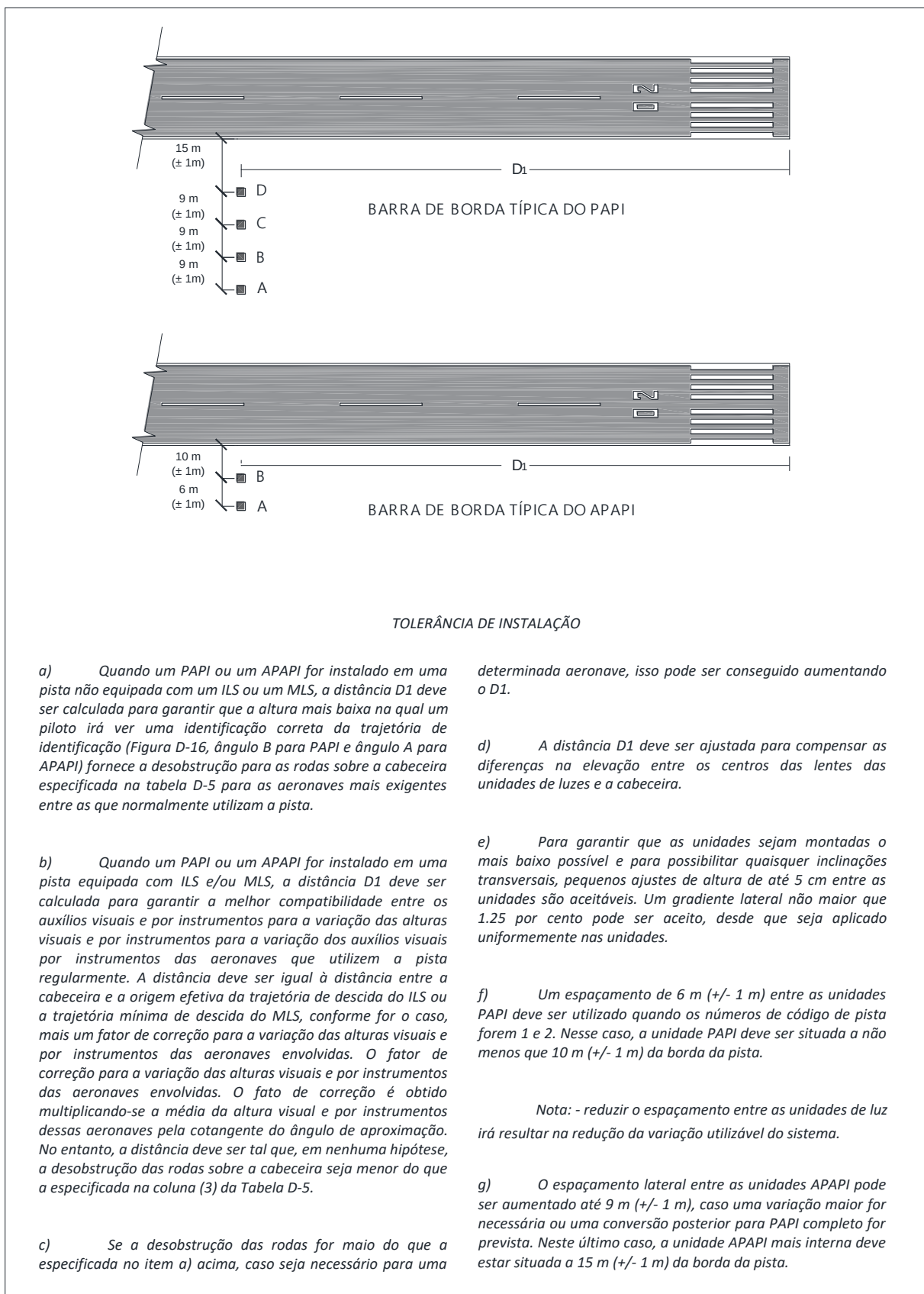
Figura D-15. Localização do PAPI e do APAPI
