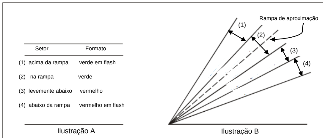
Figura 155.347-1 - Formato do sinal HAPI
