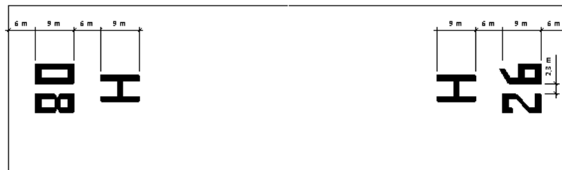
Figura 155.305-1 - FATO tipo pista de pouso e decolagem: exemplo de sinalizações horizontais de identificação de heliponto e designação de FATO.
