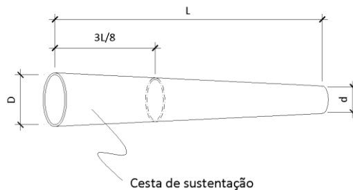
Figura 155.301-1 - Dimensões do cone de vento.
