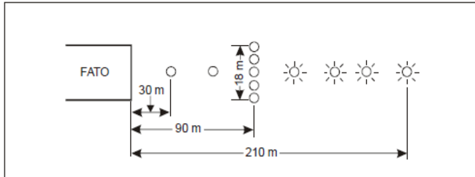
Figura 155.341-1 - Sistema de luzes de aproximação
