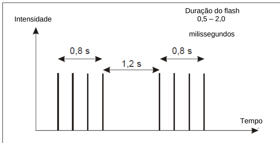
Figura 155.339-1 - Características do flash do Farol de Heliponto
