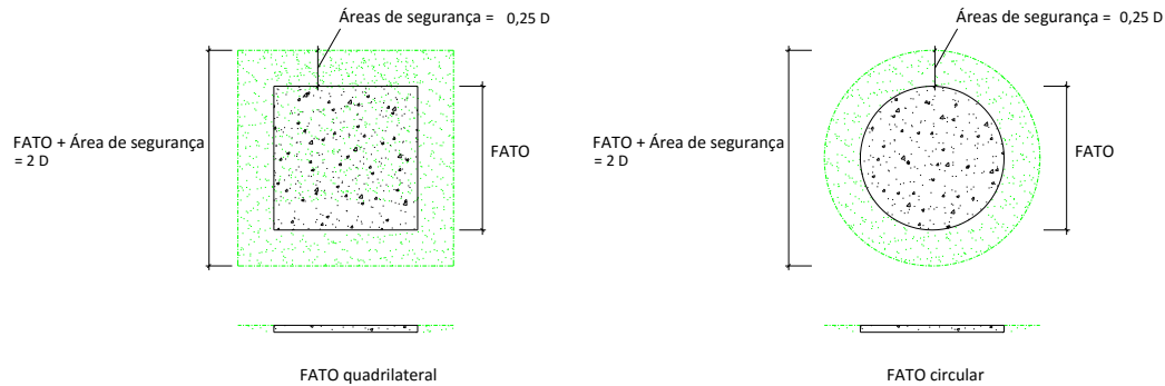
Figura 155.209-1 - FATO e área de segurança associada.
