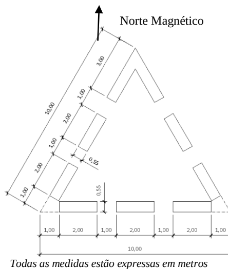
Figura 155.319-1 - Sinalização horizontal de ponto de visada de heliponto
