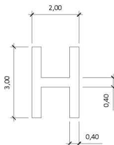
Figura 155.303-1 - Sinalização horizontal de identificação de heliponto.
