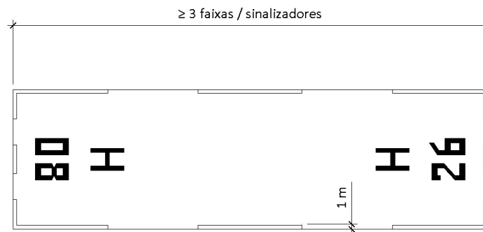
Figura 155.315-1 – Sinalização horizontal de perímetro de FATO tipo pista de pouso e decolagem.
