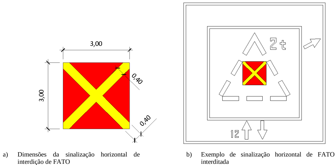
Figura 155.335-1 – Sinalização horizontal de interdição de FATO.
