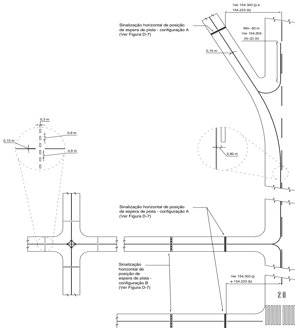
Figura D-6. Sinalização horizontal de pista de táxi (exibida em conjunto com a sinalização horizontal básica de pista de pouso e decolagem)
